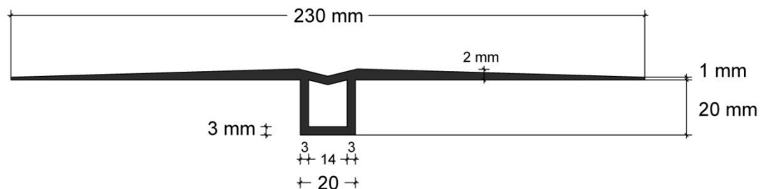
1.Sectiunea Serviseal B scara 1 : 10
